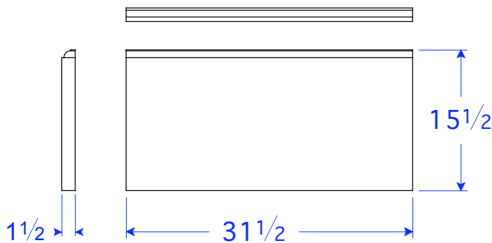
BM 14-1.5x15 STR 15 1/2"H x 31 1/2"L x 1 1/2"T
