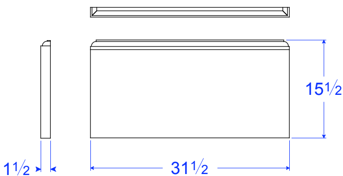
BM 14-1.5x15.5 DR 15 1/2"H x 31 1/2"L x 1 1/2"T
