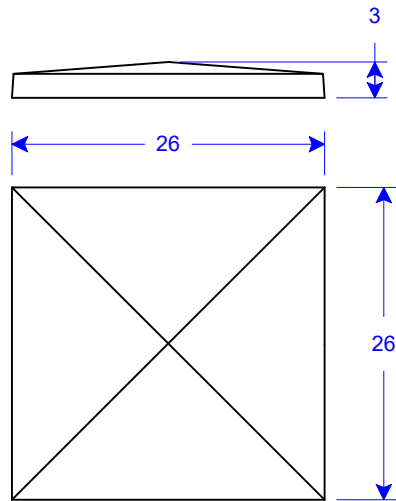
PC 13-26 P3 26"W x 26"L x 3"H
