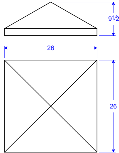
PC 13-26 P9.5 26"W x 26"L x 9 1/2"H
