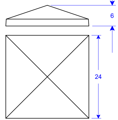
PC 13-22 P6 24"W x 24"L x 6"H
