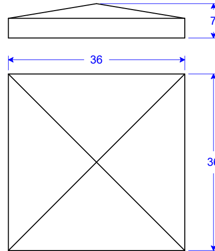
PC 13-36 P7 36"W x 36"L x 7"H
