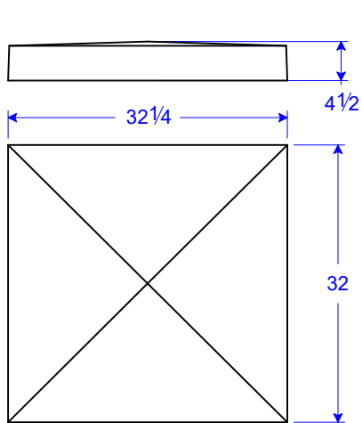
PC 13-32 P4.5 32"W x 32"L x 4 1/2"H
