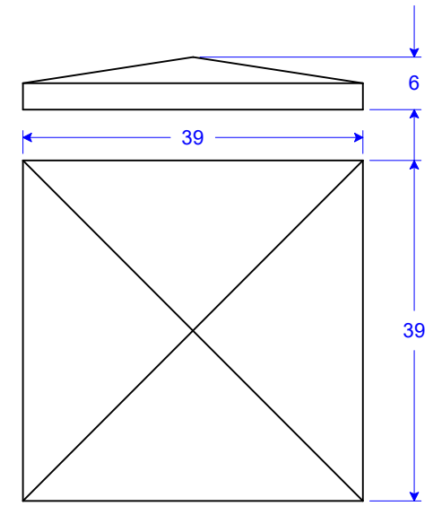
PC 13-39 P6 39"W x 39"L x 6"H
