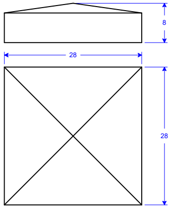
PC 13-28x28 P8 28"W x 28"L x 8"H
