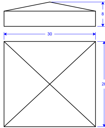
PC 13-28x30 P8 28"W x 30"L x 8"H
