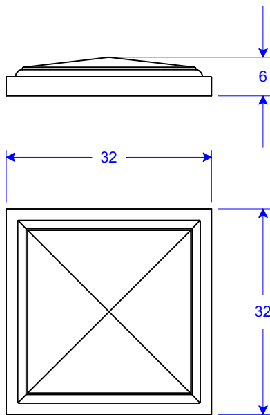
PC 19-32 P6 32"W x 32"L x 6"H
