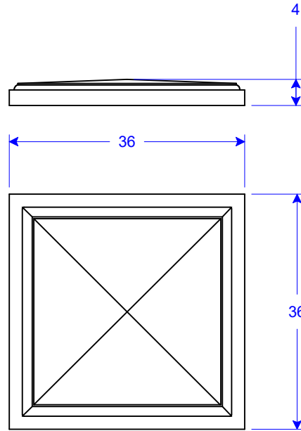
PC 19-36 P4 36"W x 36"L x 4"H
