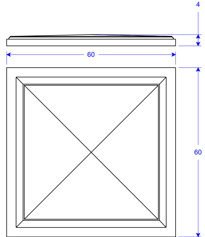
PC 19-60 P4 60"W x 60"L x 4"H
