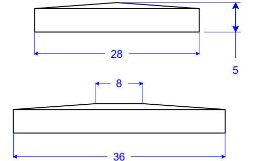
PC 20-28x36 P5 28"W x 36"L x 5"H
