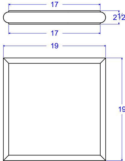
PC 31-19 BNF 17"W x 17"L x 2 1/2"H
