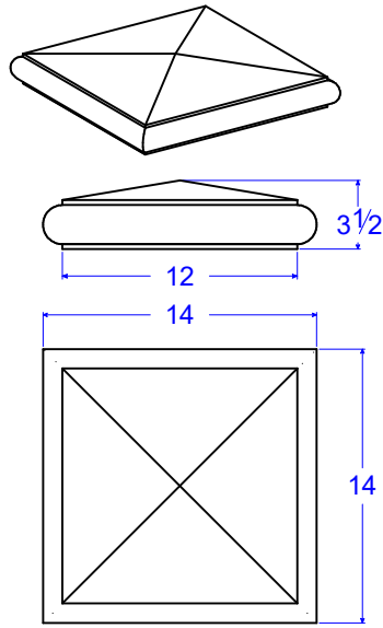
PC 31-14 BN P3.5 12"W x 12"L x 3 1/2"H
