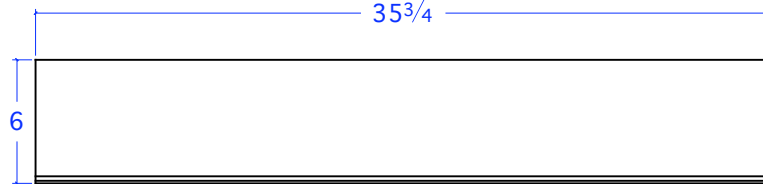
SM 19-6x3.25 STR L 3 1/4"W x 35 3/4"L x 6"H
