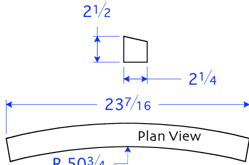
SM 27-2.25x2.5 STR R 45 1/2 2 1/4"W x 23 7/16"L x 2 1/2"H
