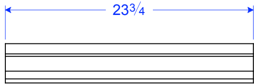
TM 26-2M STR 4 3/4"W x 23 3/4"L x 3 3/4"H
