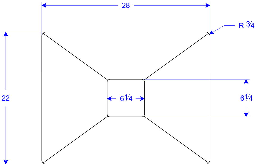
PC 01-22 P4.5 22"W x 28"L x 4 1/2"H
